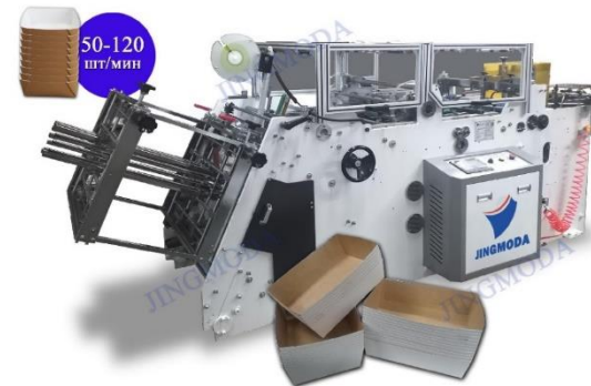
Оборудование для производства бумажной одноразовой упаковки для продуктов JMD-DU800
